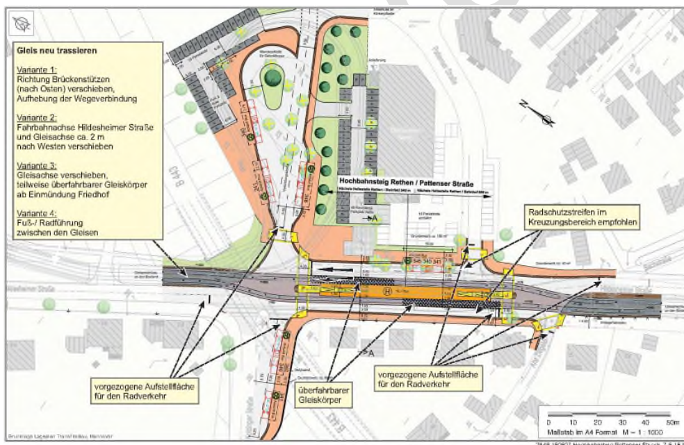
Abb. 2.1: Konzept für Umsteigestation Rethen / Pattenser Straße (Quelle: TransTecBau und Infra 2016 mit Anmerkungen PGT zu ergänzenden Maßnahmen)
