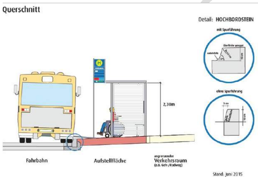
Abb. 2.5: Schnitt: Muster-Bushaltestelle (Region Hannover 7 )
