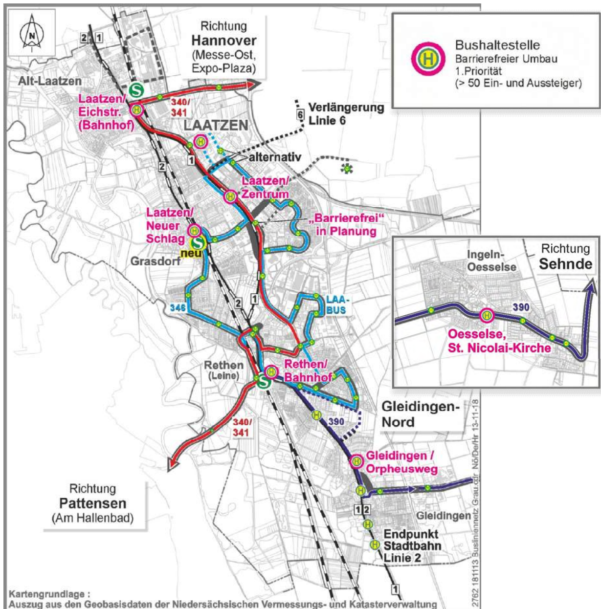
Abb. 4.1: Barrierefreier Ausbau von Bushaltestellen und S-Bahnhof Rethen empfohlen
