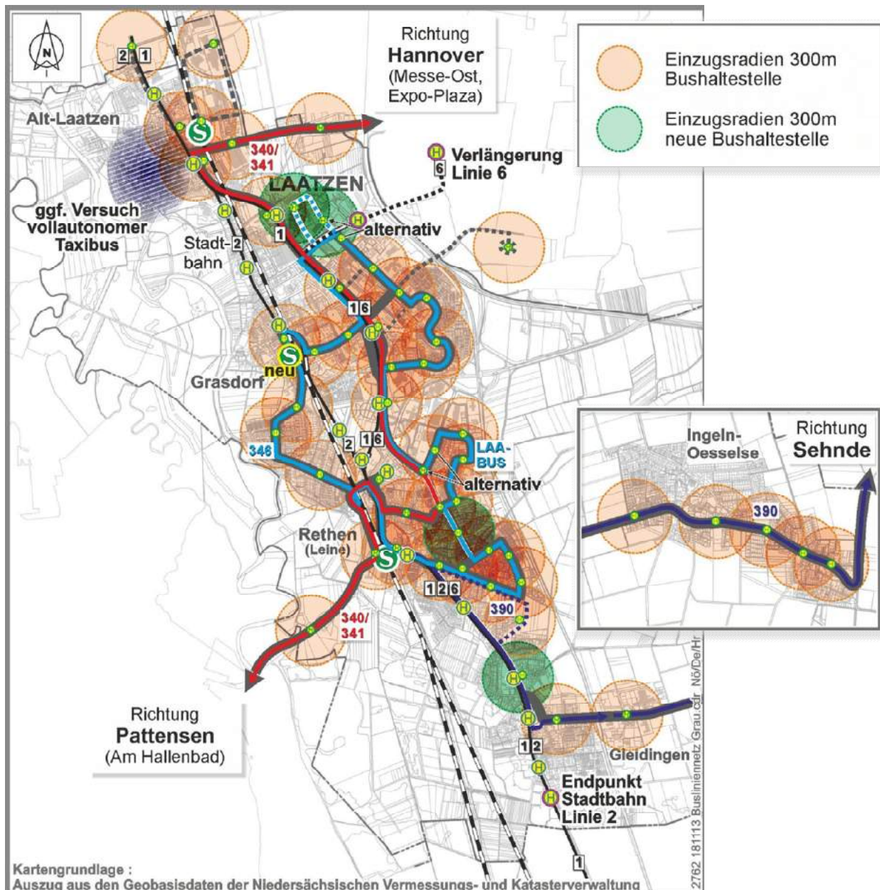
Abb. 4.7: Stadtbusroutenkonzept Laatzen mit Einzugsradien
